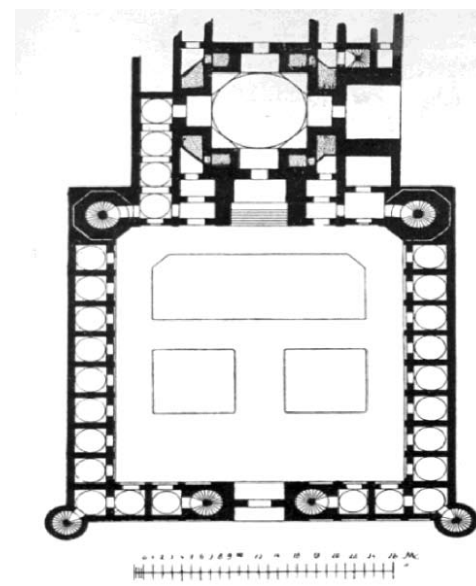
صورة ٢٤٣: رسم تخطيطي لمدرسة تيلليه كاري في سمرقند (نقلًا عن جريدة البناء العامة ١٨٩٨)
