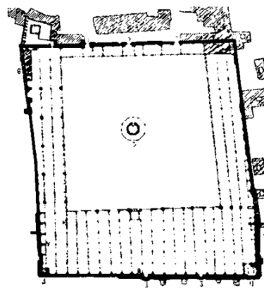
الصورة ٣٩٢: رسم تخطيطي لمسجد عمرو في القاهرة (نقلًا عن فرانز باشا) لإبراز التناسب بمبنى المسجد فإن الرسم التخطيطي يظهر هنا على قدر المستطاع في نفس الاتجاه (الإيوان بالجهة السفلى) لذا ظهرت العلامات المذكورة بالمقلوب ولكن هذا ليس له أهمية.
