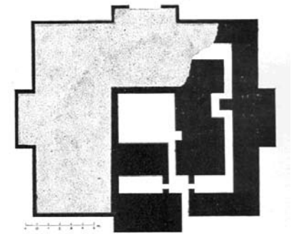
صورة ٢٧٤: الأساسات أسفل الأرض للفنار العربي القلعة بشرق الجزائر (نقلاً عن صلاح الدين ، الآثار العربية في قلعة بني حماد)
