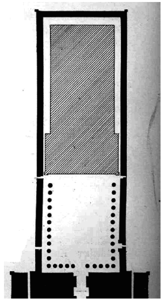
الصورة ٣٨٨: رسم تخطيطي لمعبد إدفو (نقلاً عن بيديكير)
