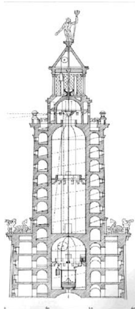
صورة ٧١: مقطع عرضي للفاروس، مع توضيح للآلة المائية وتشبيد المرأة. افتراض
