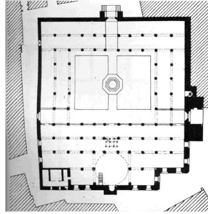
الصورة ٤١٩ : مسجد المارداني بالقاهرة (نقلًا عن لجنة حفظ الآثار العربية)
