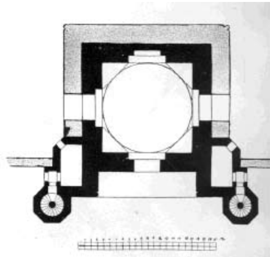
صورة ٢٥٠: رسم تخطيطي لمسجد في مدرسة بيبي غانم بسمركند ( نقلاً عن جريدة البناء العامة ١٨٩٨ )
