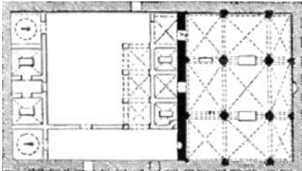
صورة ٩١: الرسم التخطيطي للحرم في حبرون نقلاً عن كوندرا (فيرجسون، تاريخ العمارة القيّمة والعصور الوسطى (١١)
