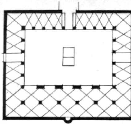
الصورة ٤٢١ : المسجد الكبير بطرابلس (نقلًا عن فاتيو)
