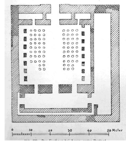
صورة ٤٠٠ : مبنى الاحتفال في آشور. المرحلة الأولى
