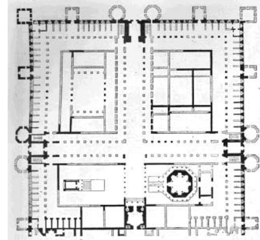
الصورة ٤٤٠: الجزء الشمالي من القصر الإمبراطوري في سبلاتو في سمرقند (نقلًا عن فيرجوسون، تاريخ العمارة القديمة والعصور الوسطى، ١)
