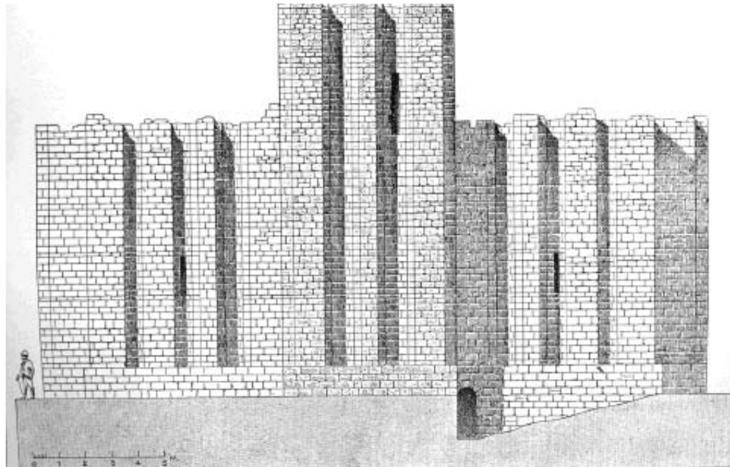
صورة ٢٧٢: منظر للفتار العربى القلعة بشرق الجزائر (نقلًا عن صلاح الدين ، الآثار العربية في قلعة بني حماد)
