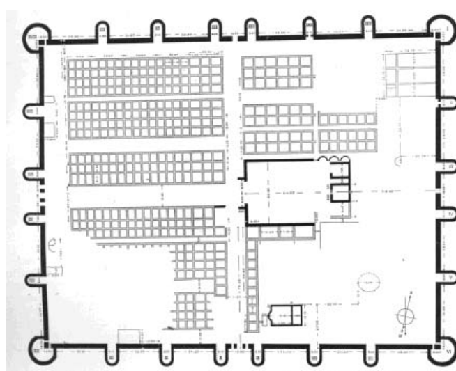
الصورة ٤٣٢: المعسكر الروماني اللجون (نقلًا عن برونو وفيكتور درماشيسكي، الأقاليم العربية، الجزء الثاني)
