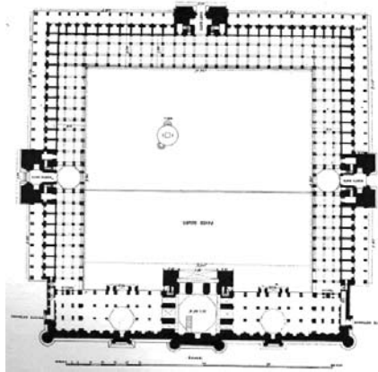
الصورة ٤١١: مسجد اطلالة بجنوب المسح الأثري في لهند)
