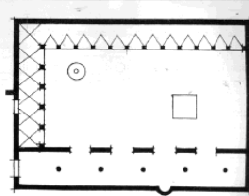
الصورة ٤٢٢ : مسجد حمص (نقلًا عن فاتيو)
