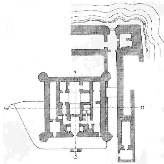
صورة ٦٨: قلعة قايتباي بممر النفق بطول الجانب الشرقي. رسم تخطيطي نقلا عن فيبر ١٩٠٦
