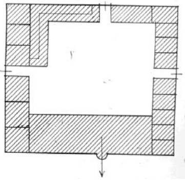
الصورة ٤٠٩: المرحلة الثانية (رسم تخطيطي للبناء)
