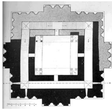
صورة ٢٧٣: رسم تخطيطي لفنار عربي القلعة بشرق الجزائر (نقلاً عن صلاح الدين ، الآثار العربية في قلعة بني حماد)
